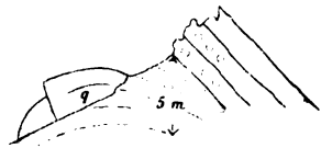
Fig. 5. Biegungen im Glimmerquarzit am Contact beim Gstellhorn
